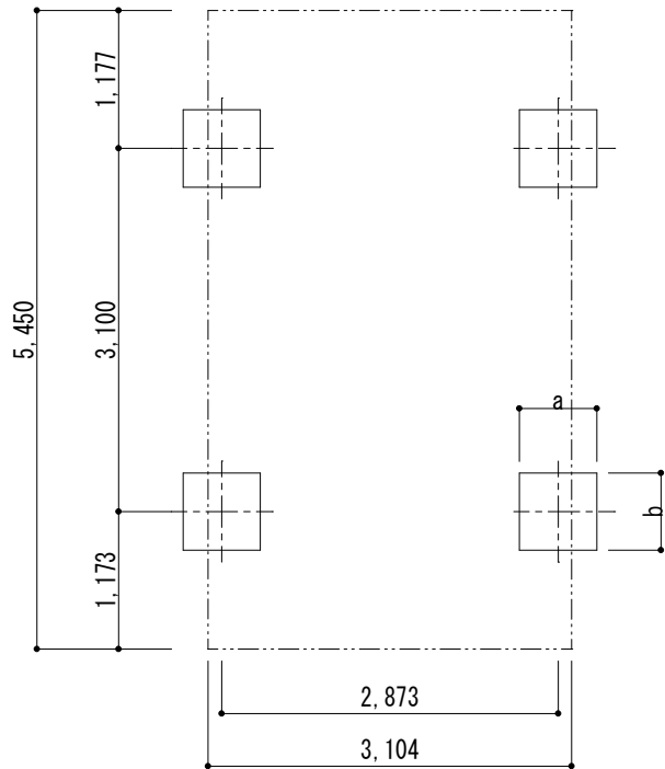
■基礎配置図
